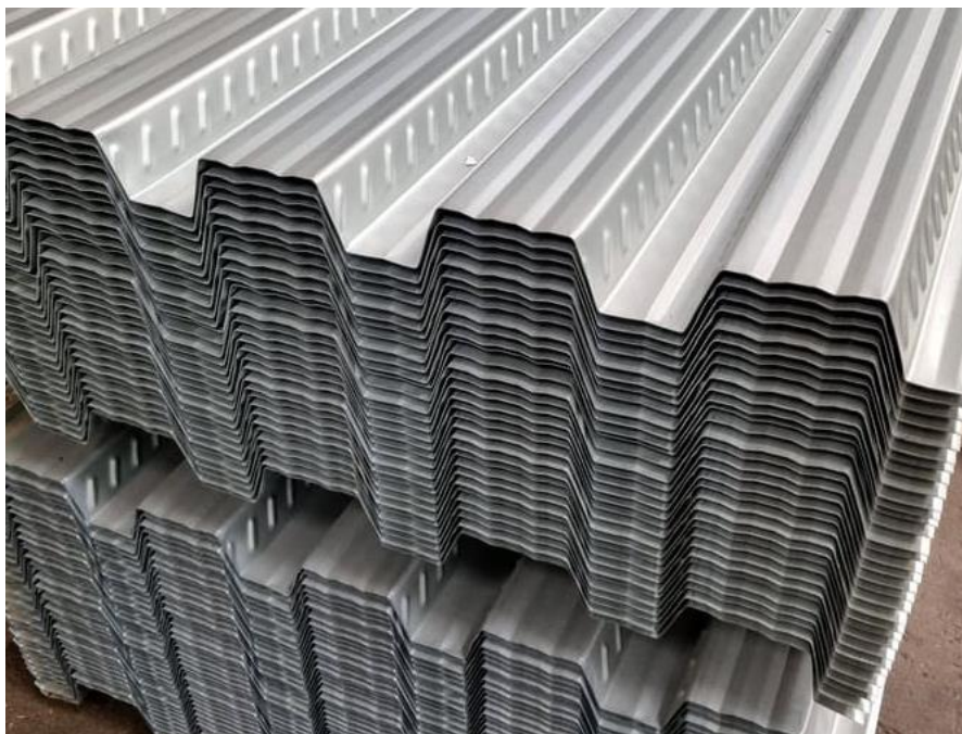
Cofraplus 60
